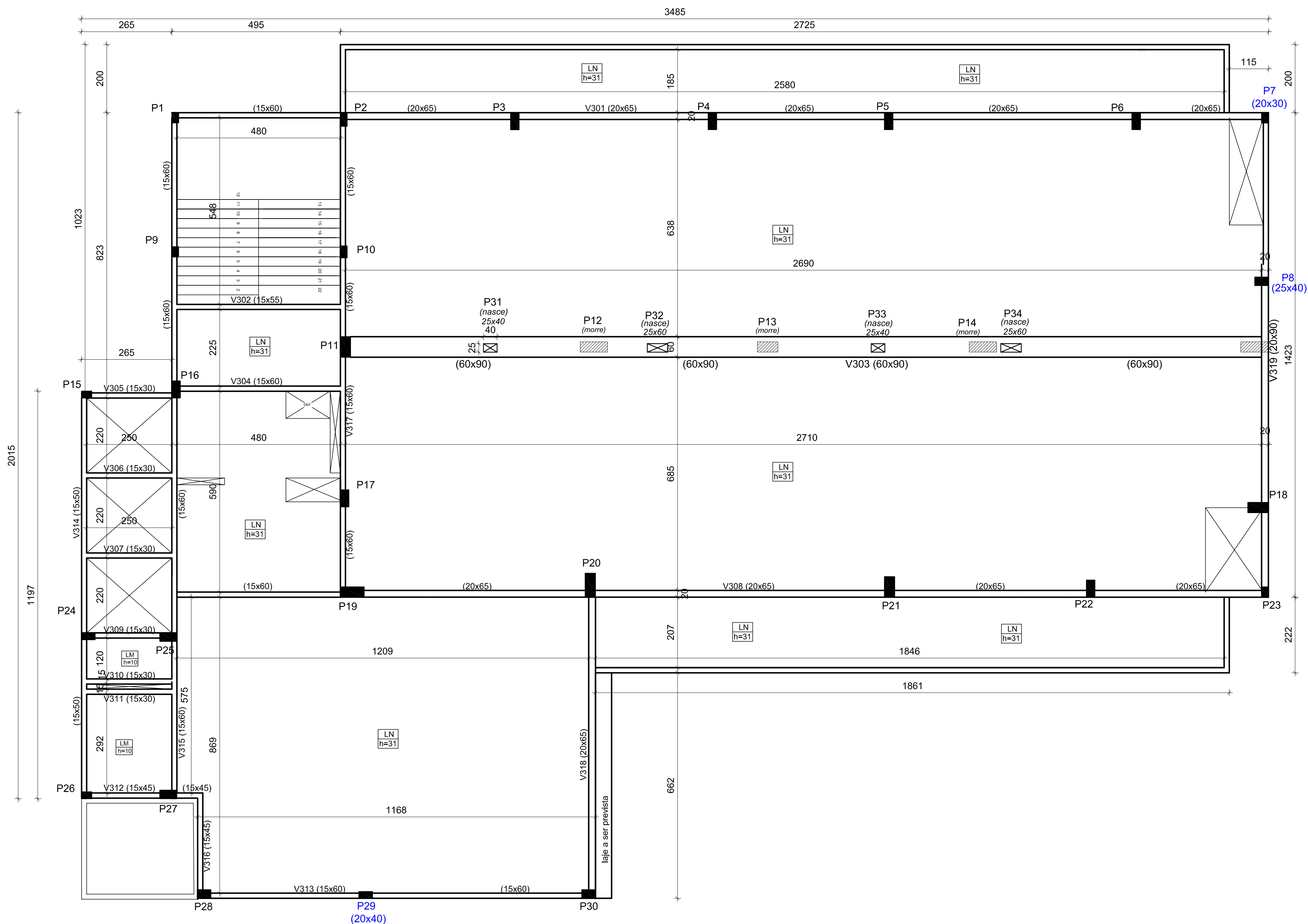
Planta de Fôrmas - 4º Pavimento Escala 1:50
